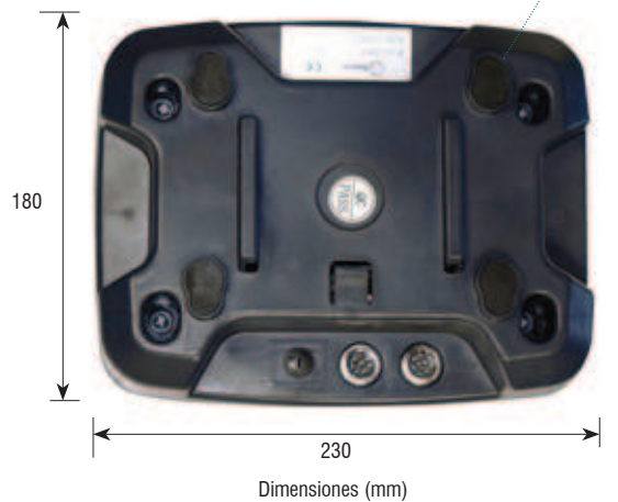
Dimensiones (mm)
